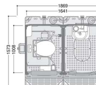
ポンプ式簡易水洗 TU-CTWiXF4
